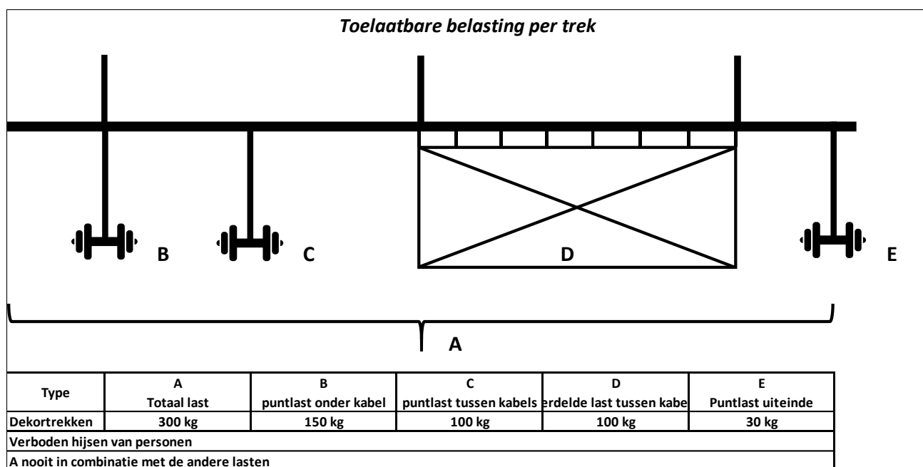
Figure 1: Lastentabel trekken
